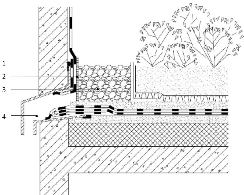
图 C.7 女儿墙泛水构造做法图
