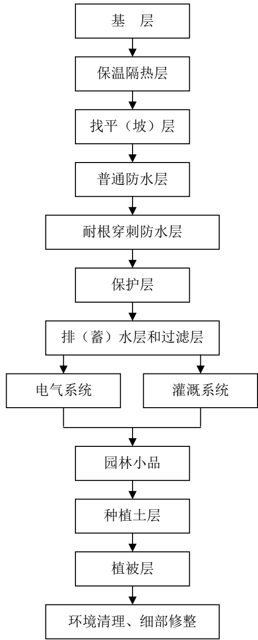
图 C.12 新建建筑屋顶绿化施工工艺流程图
