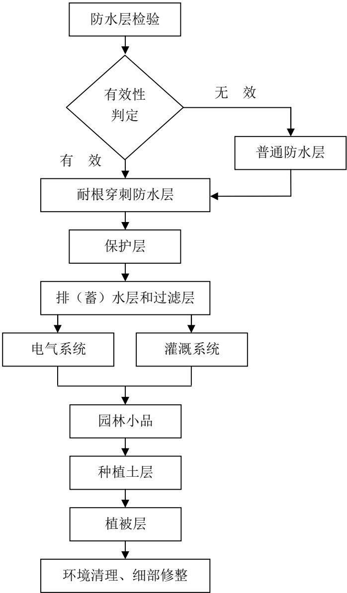
图 C.13 既有建筑屋顶绿化施工工艺流程图
